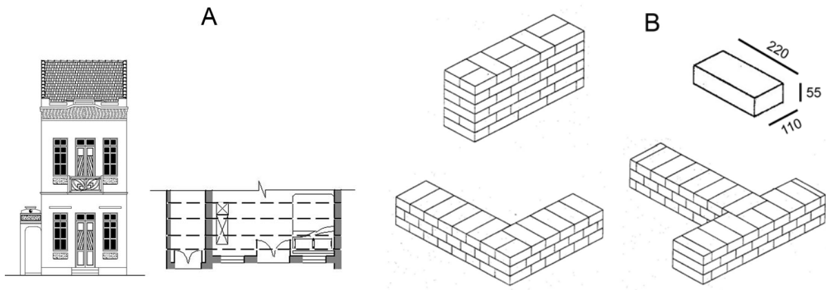
Hình 3. Ví dụ về biện pháp & vật liệu xây dựng truyền thống cho mặt đứng
