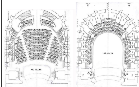
Mặt bằng khu vực sân khấu nhà hát lớn Hà Nội
