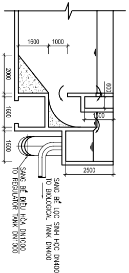
MẶT CẮT - SECTION B-B
