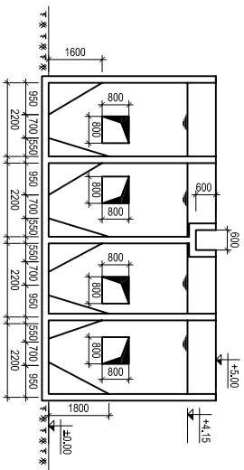
MẶT CẮT - SECTION A-A
